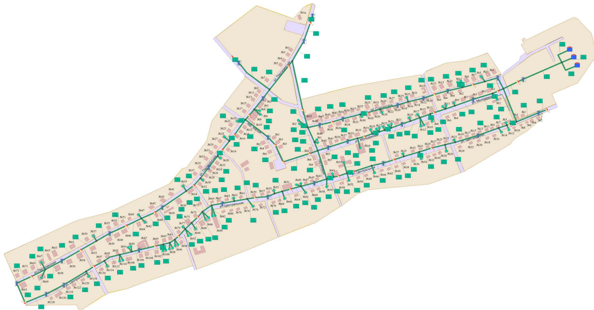
Рисунок 6.2 - Планируемая схема водопроводной сети с. Зюзя
