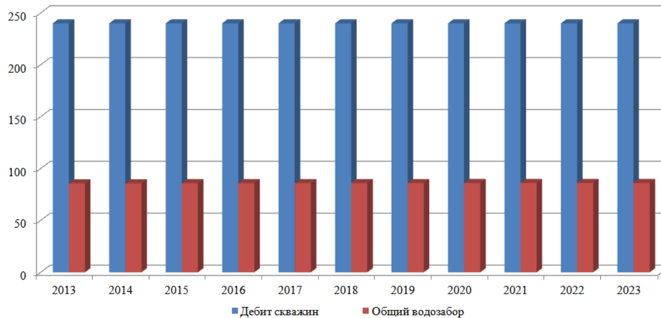
Рисунок 5.4 - Дебит скважин
