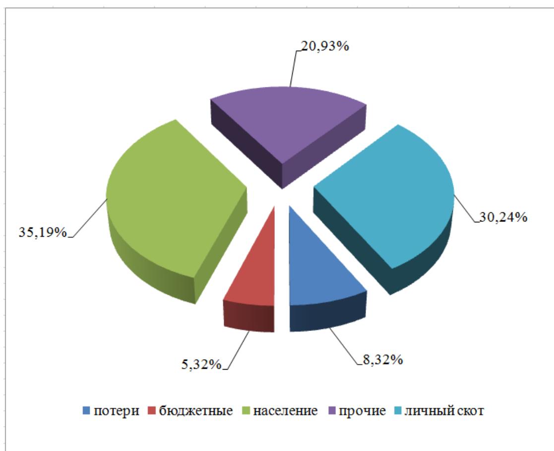
Рисунок 5.1 - Баланс водоснабжения д. Казанцево
