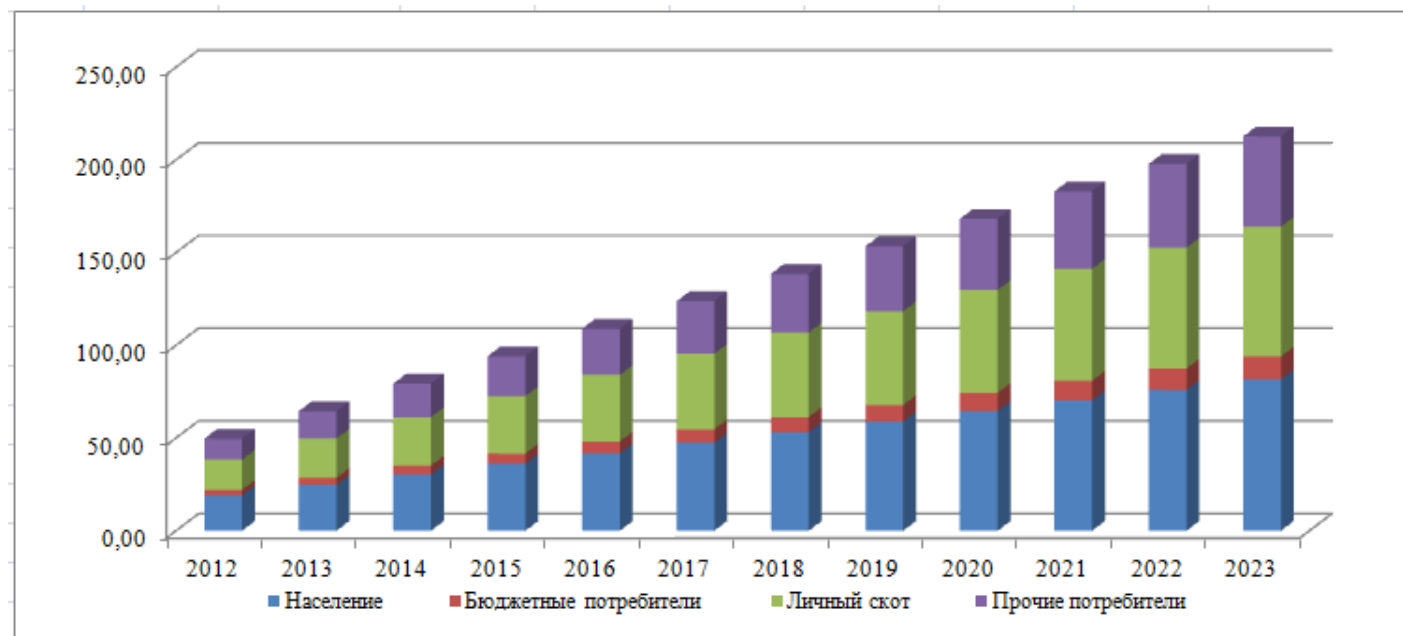
Рисунок 5.2 – Перспективное водопотребление с разбивкой по группам потребителей
