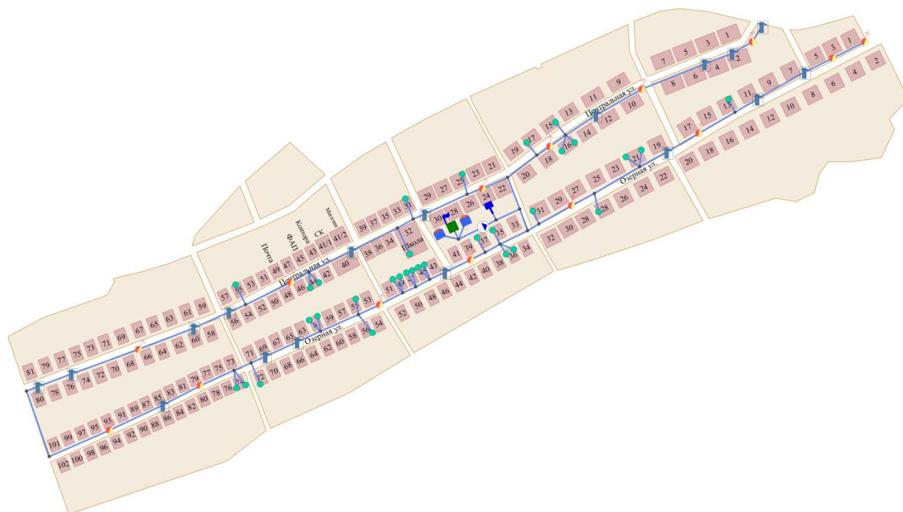
Рисунок 2.1 - Зона действия централизованного водоснабжения д. Казанцево
