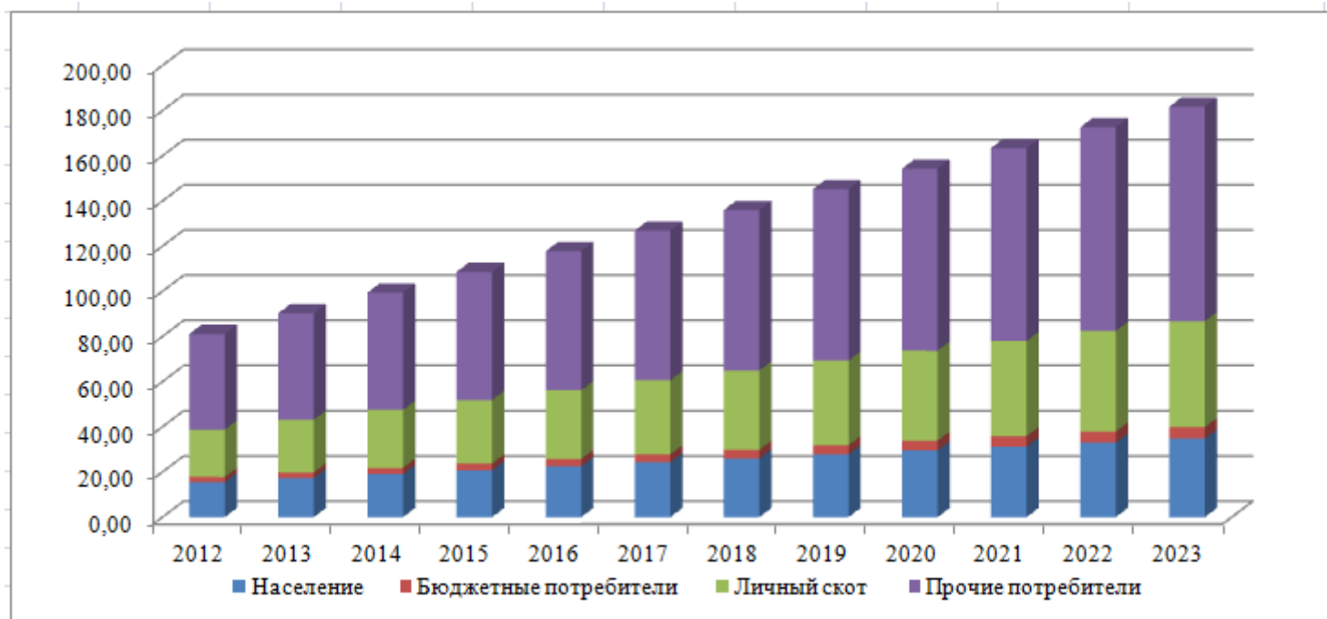
Рисунок 5.2 – Перспективное водопотребление с разбивкой по группам потребителей
